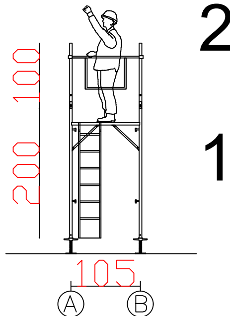
ELEVACION EJE 2
